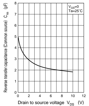
C_{rss} - V_{DS}
